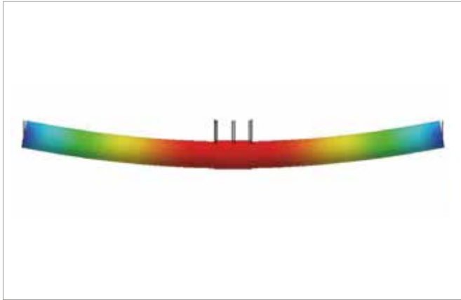
힘인장강도 해석
