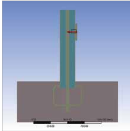
3차원 해석모델
